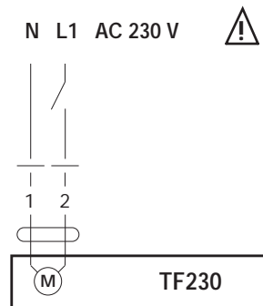
接线图 单线控制
