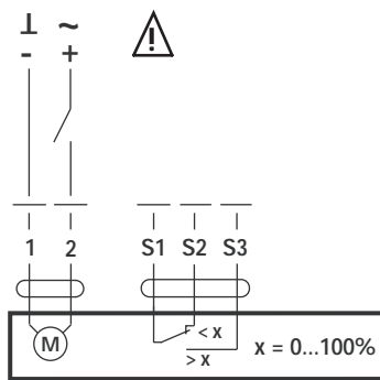
接线图 单线控制
