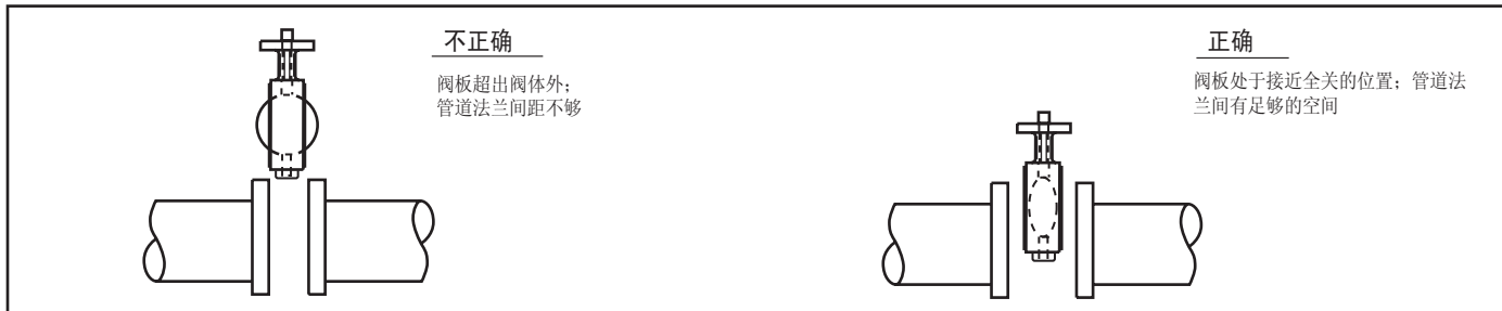
图2: 阀门对中
