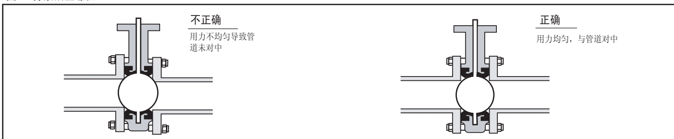
图3: 拧紧法兰螺栓
